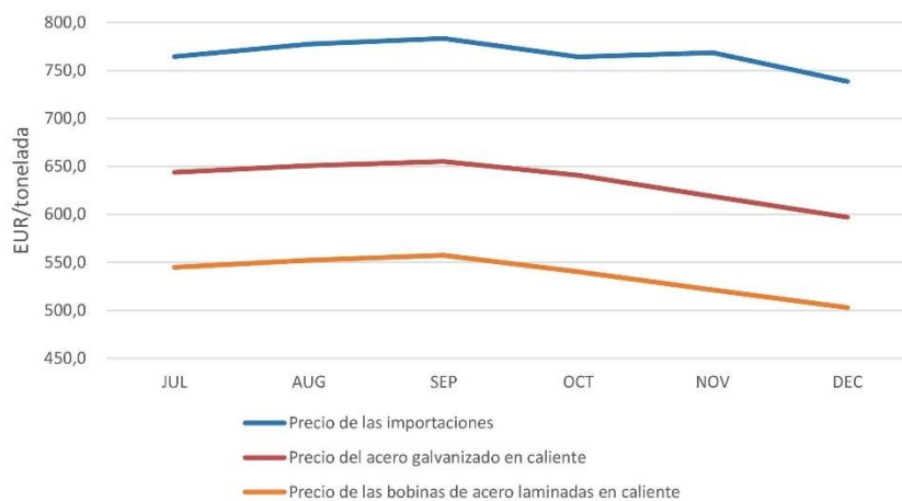
Gráfico 4: Precios de importación del acero galvanizado en caliente y las bobinas de acero laminadas en caliente en el segundo semestre de 2018
